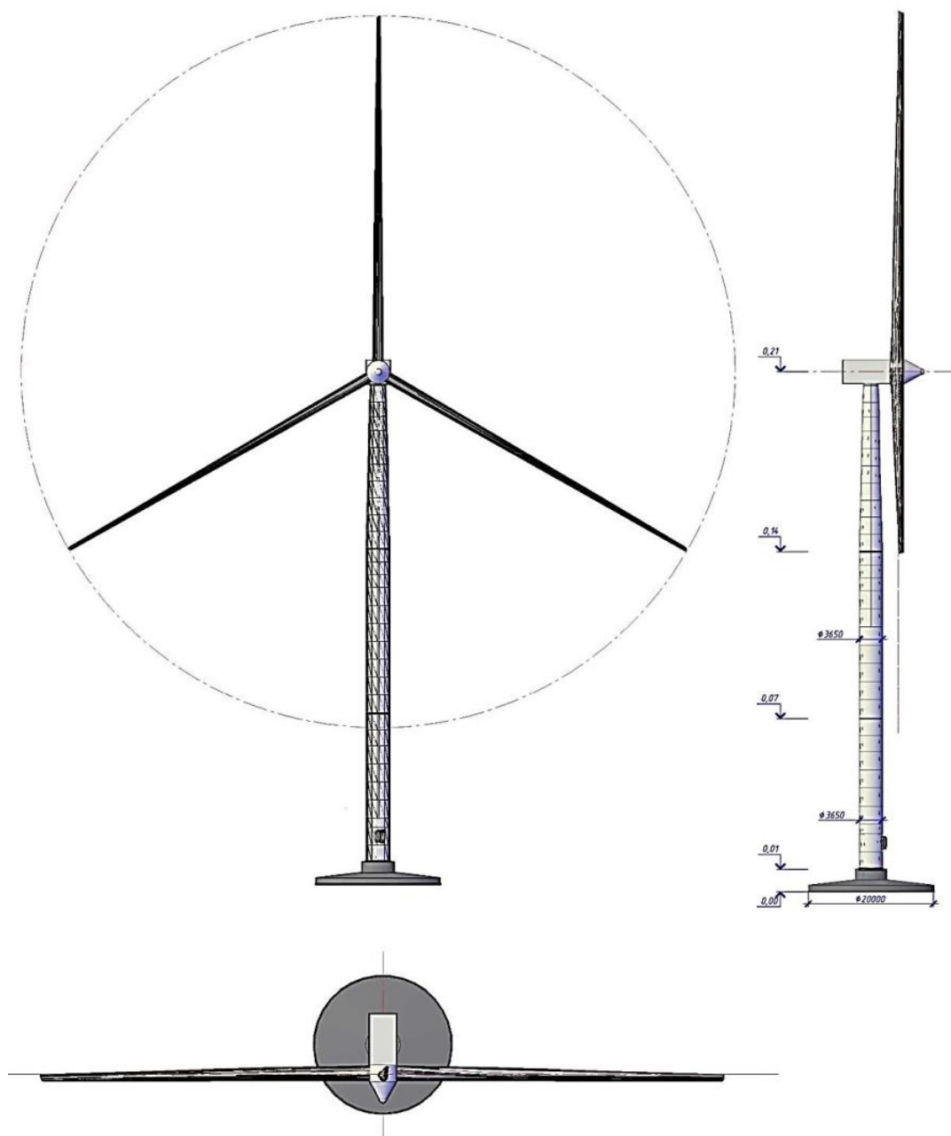
Рисунок 2.6 Общий вид ВЭУ «Enercon E6618/7085»
