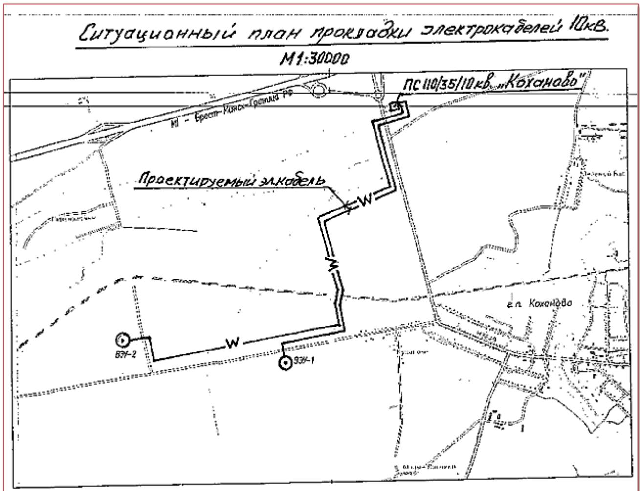
Рисунок 2.8 – Ситуационный план прокладки электрокабелей 10 кВ
