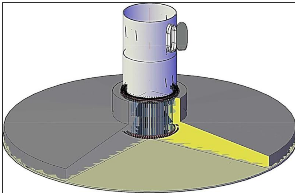
Рисунок 2.7 Общий вид фундамента ВЭУ1 и ВЭУ2
